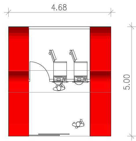
draufsicht
